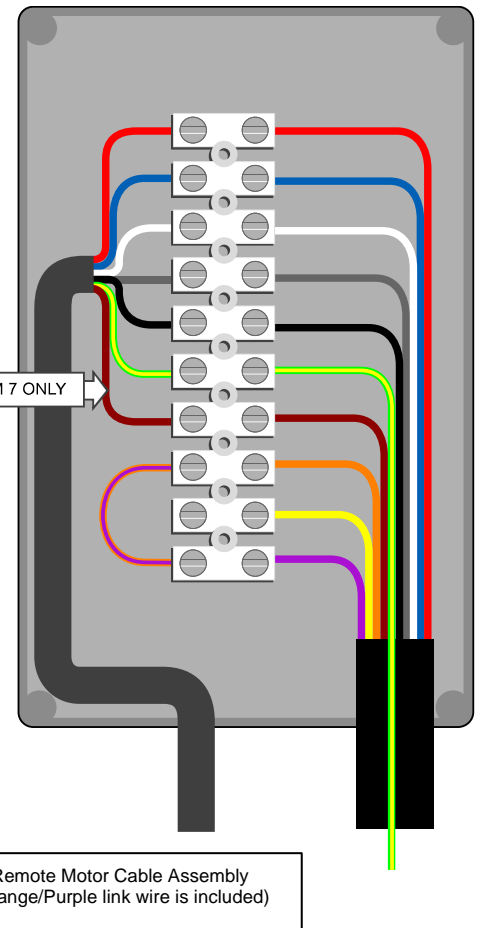
Fig. 4 SEM 7 / SEM 8 Electrical Connections
